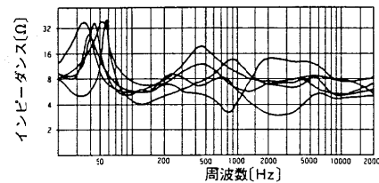
図1. 各種スピーカのインピーダンス周波数特性
