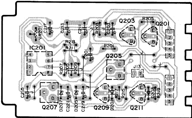
H 電流ドライブ アンプ基板 (Lch)
