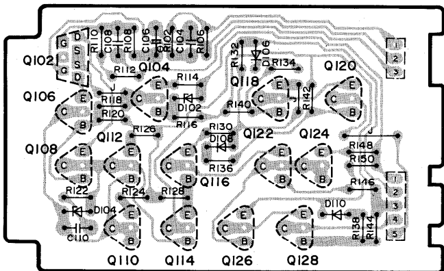
F Aクラス 電圧コントロールアンプ基板 (Rch)
