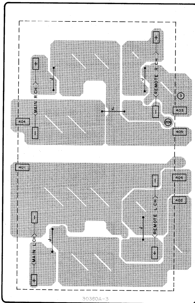
K スピーカ端子基板
