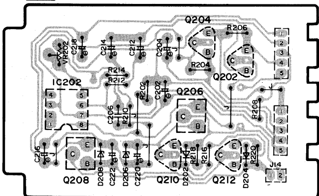
E 電流ドライブ アンプ基板 (Rch)
